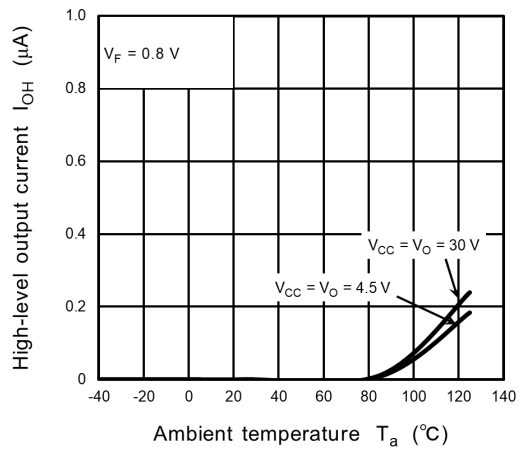
Fig. 12.2.4 I_{OH} - T_a
