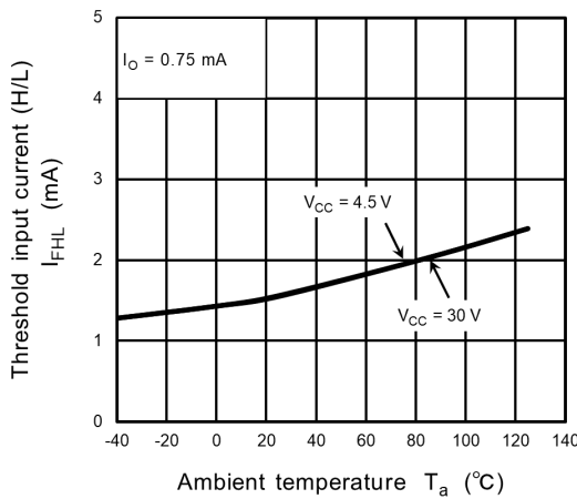
Fig. 12.2.3 I_{FHL} - T_a
