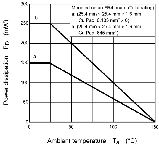
Fig. 7.3.1 P_D - T_a
