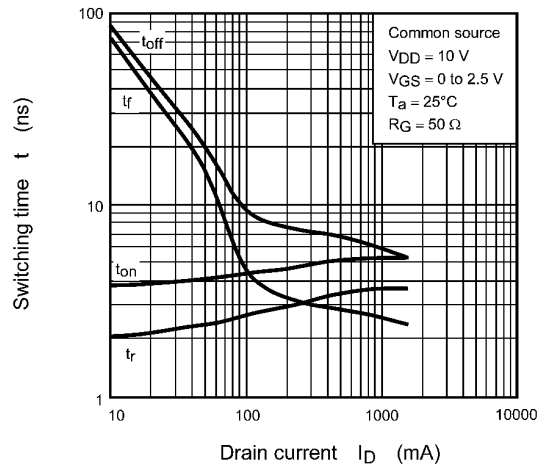
Fig. 7.1.10 t - I_D
