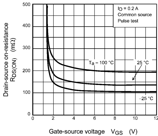
Fig. 7.1.3 R_{DS(ON)} - V_{GS}
