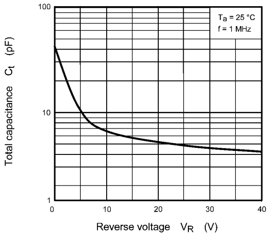
Fig. 7.2.3 C_t - V_R
