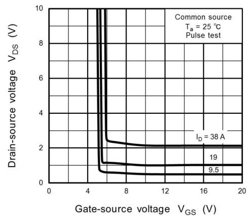
Fig. 8.4 V_{DS} - V_{GS}
