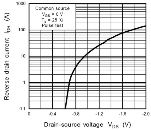
Fig. 8.8 I_{DR} - V_{DS}
