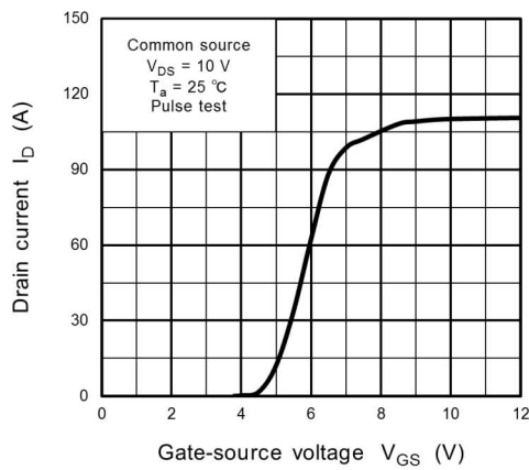
Fig. 8.3 I_D - V_{GS}
