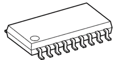
SOP18-P-375-1.27
