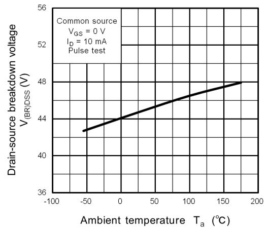
Fig. 9.12 V_{(BR)DSS} - T_a
