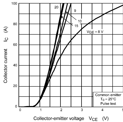
Fig. 8.2 I_C - V_{CE}
