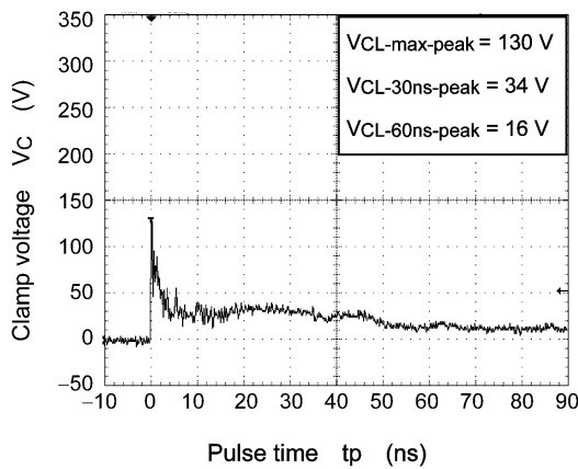
Fig. 6.1.3 +15 kV
