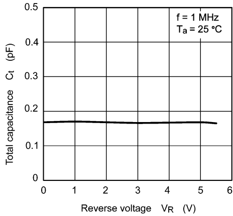
Fig. 9.3 C_t - V_R
