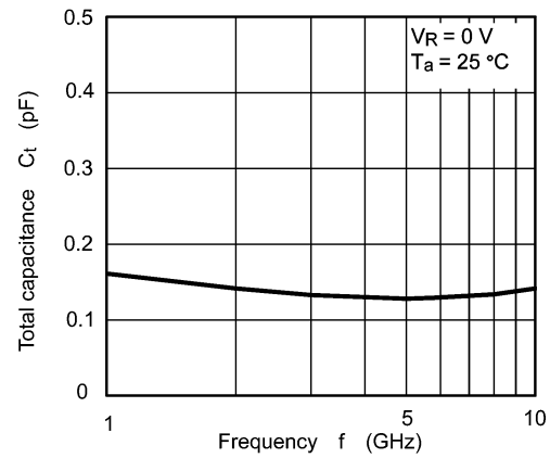
Fig. 9.4 C_t - f
