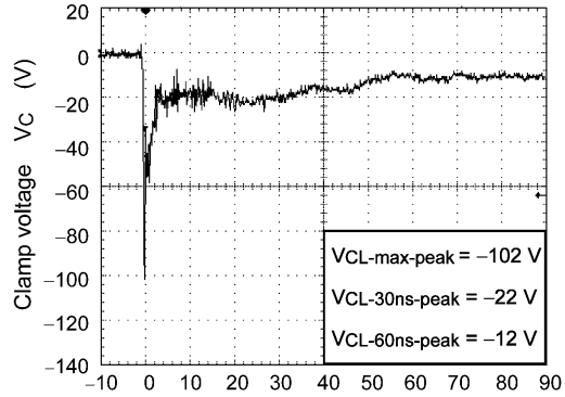
Pulse time t_p (ns) Fig. 6.1.2 -8 kV
