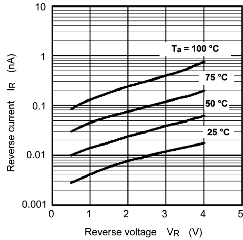
Fig. 9.2 I_R - V_R
