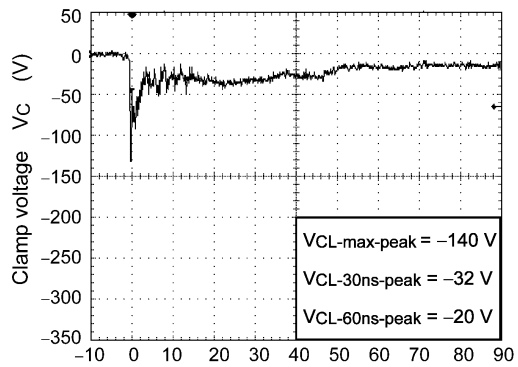
Pulse time t_p (ns) Fig. 6.1.4 -15 kV
