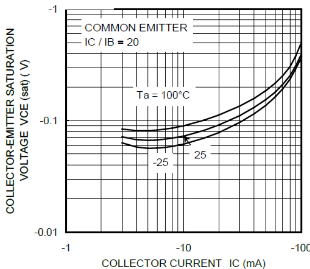
Fig. 10.17 RN2315 V_{CE(sat)}-I_C
