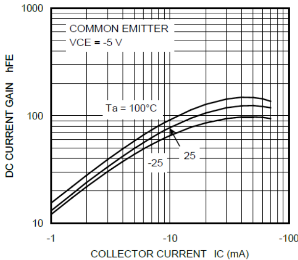
Fig. 10.15 RN2318 h_{FE}-I_C
