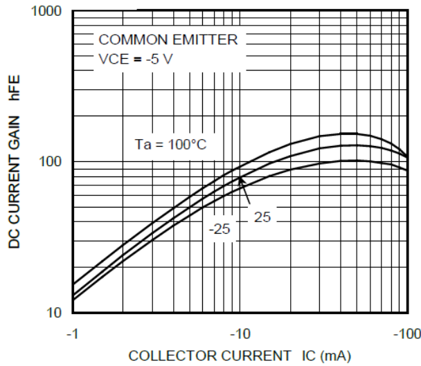
Fig. 10.13 RN2316 h_{FE}-I_C
