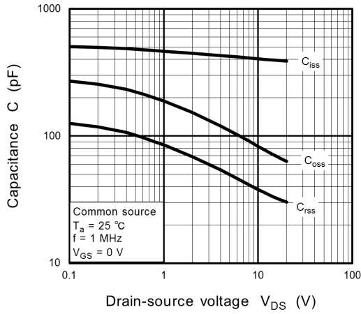
Fig. 7.7 C - V_{DS}
