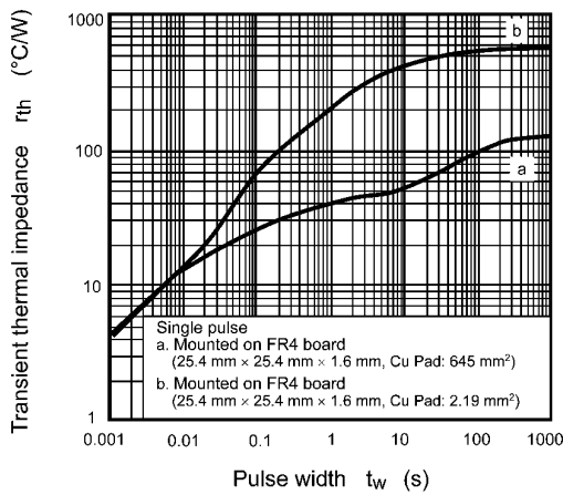
Fig. 7.11 r_{th} - t_w
