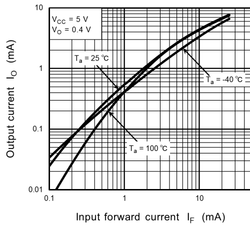
Fig. 13.2.4 I_O - I_F
