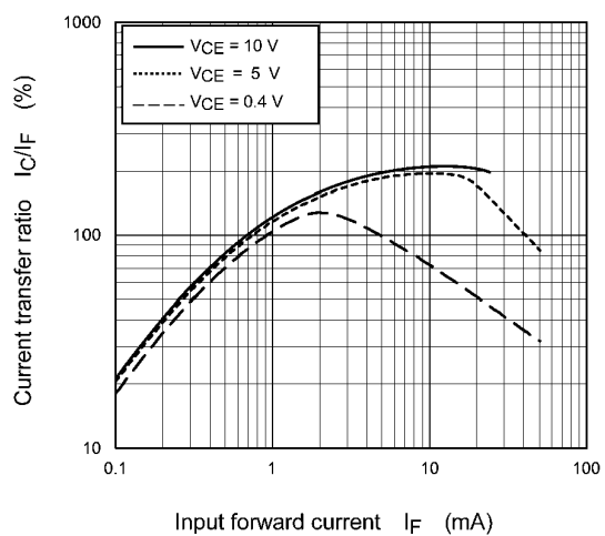
Fig. 11.12 I_C/I_F - I_F
