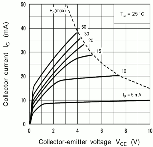
Fig. 11.7 I_C - V_{CEO}
