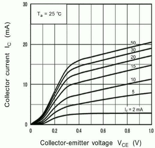
Fig. 11.8 I_C - V_{CEO}
