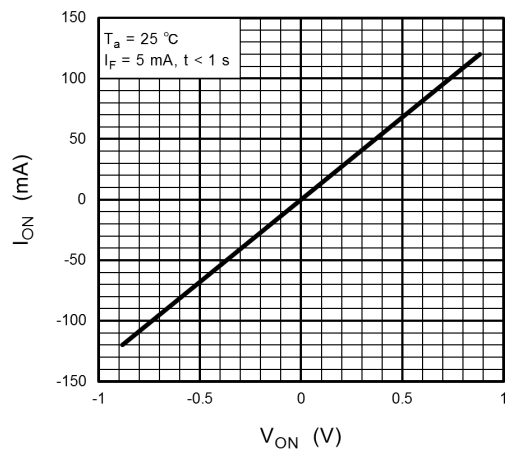
Fig. 12.4 I_{ON} - V_{ON}
