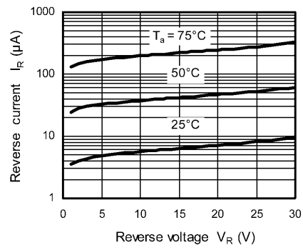
Fig. 9.2 I_R - V_R
