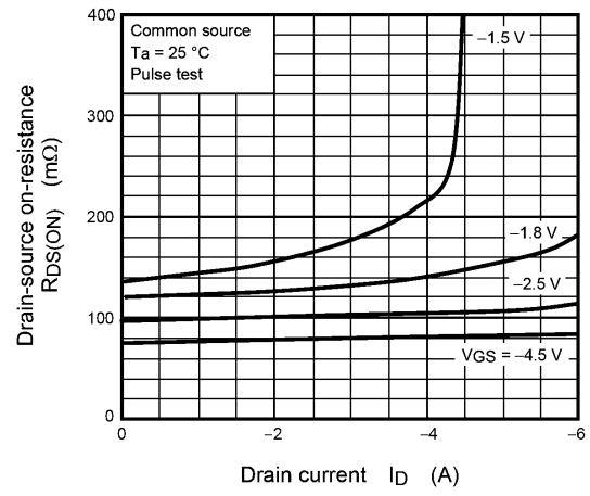
Fig. 8.4 R_{DS(ON)} - I_D
