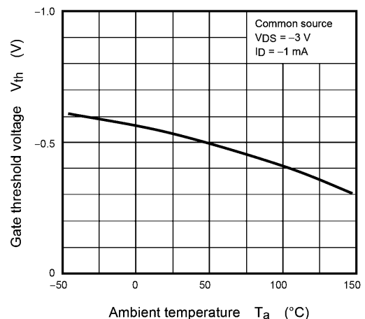
Fig. 8.6 V_{th} - T_a
