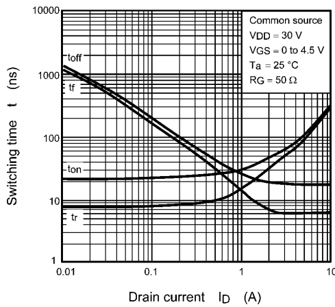
Fig. 7.9 t - I_D
