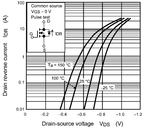
Fig. 7.7 I_{DR} - V_{DS}
