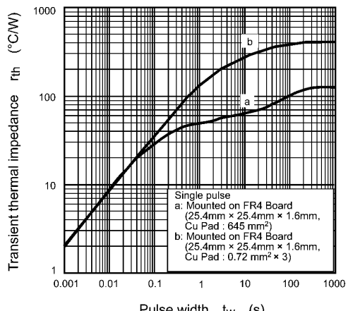
Fig. 7.12 r_{th} - t_w
