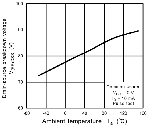
Fig. 8.7 V_{(BR)DSS} - T_a
