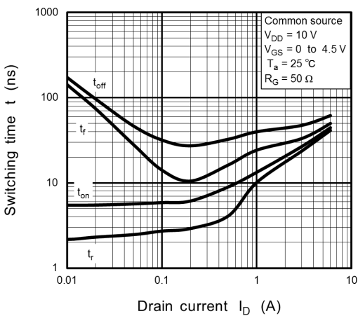
Fig. 7.9 t - I_D
