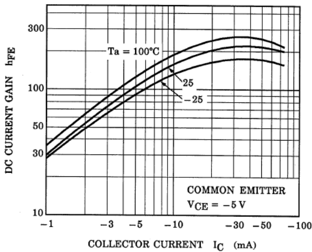
Fig. 10.15 RN2103 h_{FE}-I_C
