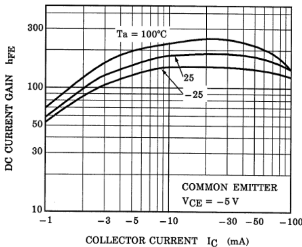
Fig. 10.17 RN2105 h_{FE}-I_C
