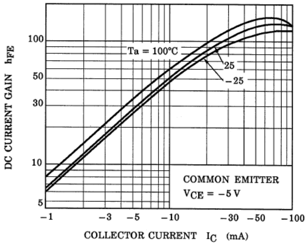
Fig. 10.13 RN2101 h_{FE}-I_C
