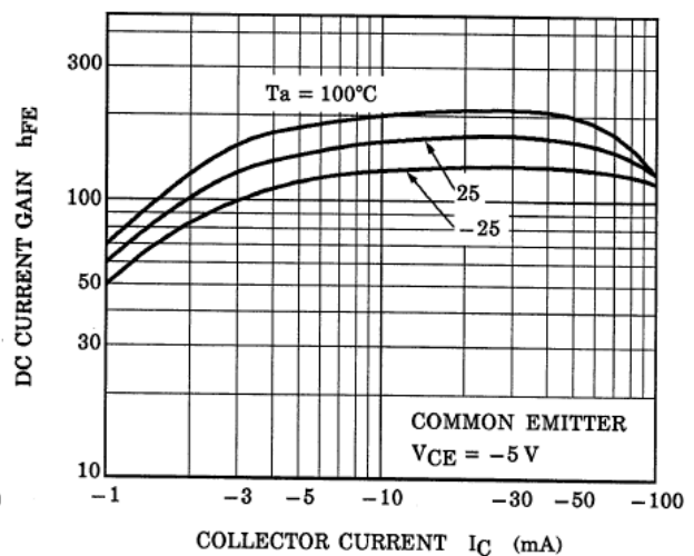
Fig. 10.18 RN2106 h_{FE}-I_C
