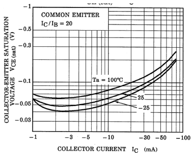
Fig. 10.21 RN2103 V_{CE(sat)}-I_C
