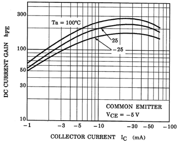
Fig. 10.16 RN2104 h_{FE}-I_C
