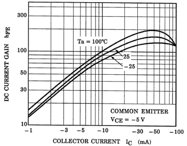
Fig. 10.14 RN2102 h_{FE}-I_C
