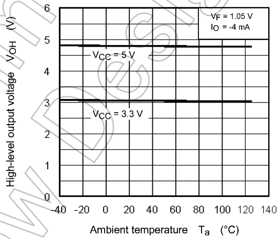
Fig. 12.2.4 V_{OH} - T_a
