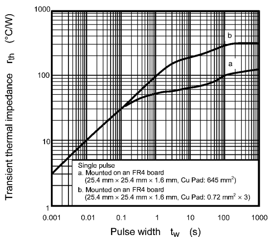
Fig. 7.11 r_{th} - t_w
