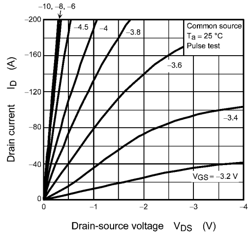
Fig. 9.2 I_D - V_{DS}
