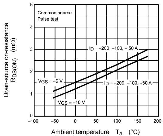
Fig. 9.6 R_{DS(ON)} - T_a
