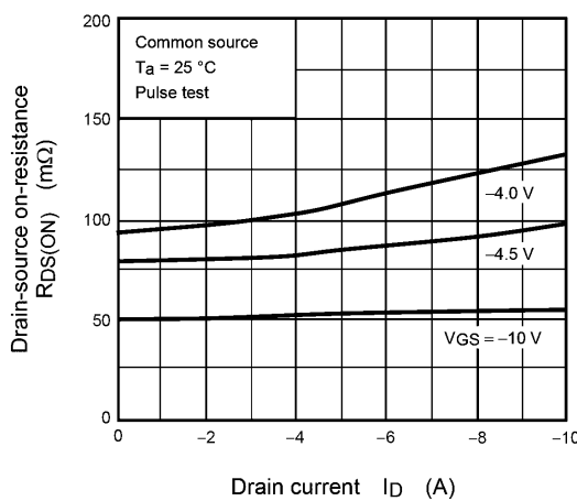
Fig. 8.5 R_{DS(ON)} - I_D
