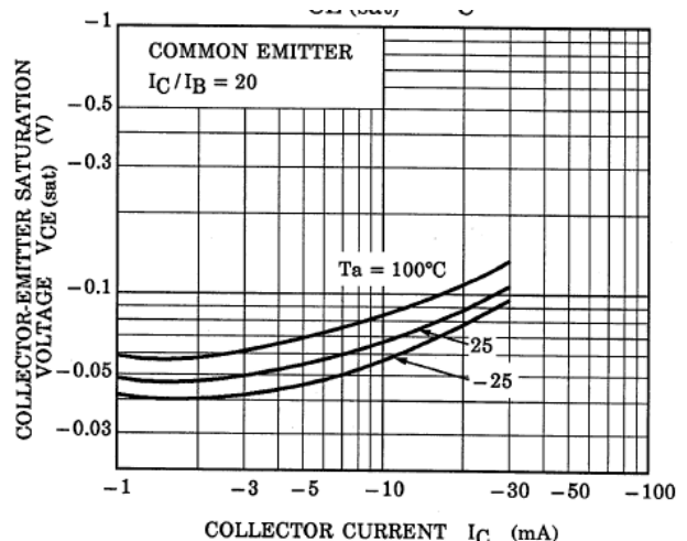
Fig. 10.22 RN2104 V_{CE(sat)} - I_C
