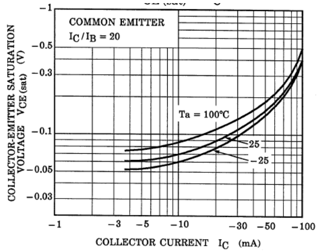
Fig. 10.20 RN2102 V_{CE(sat)} - I_C
