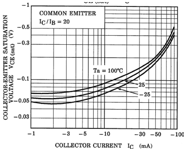
Fig. 10.23 RN2105 V_{CE(sat)} - I_C
