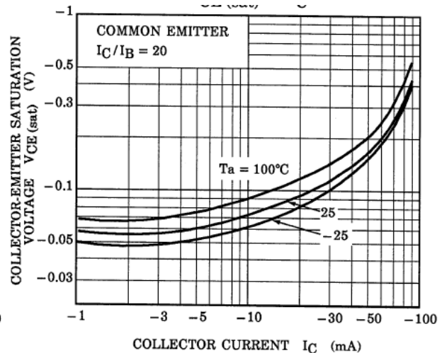
Fig. 10.24 RN2106 V_{CE(sat)} - I_C
