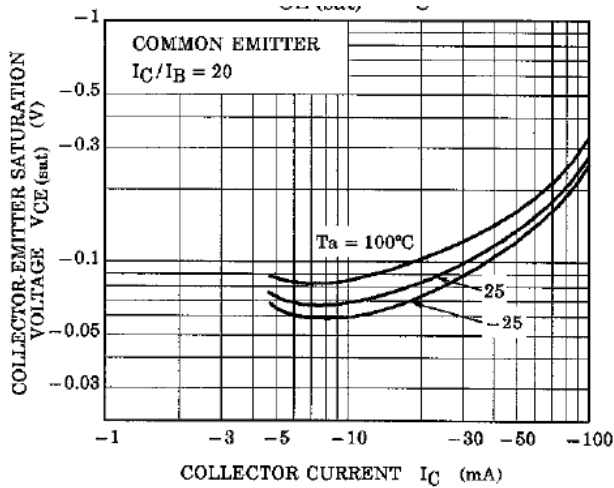
Fig. 10.19 RN2101 V_{CE(sat)} - I_C
