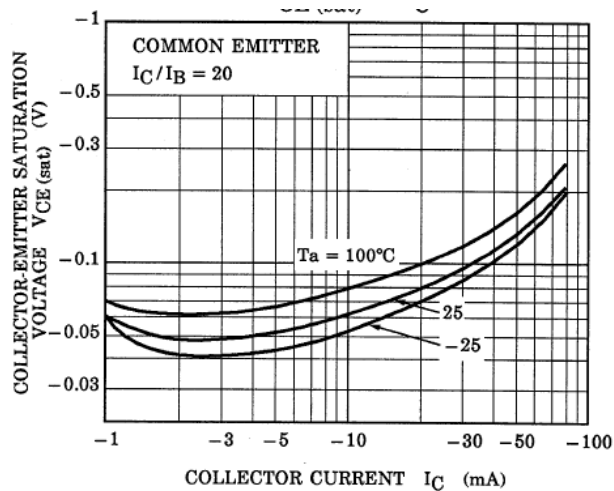
Fig. 10.21 RN2103 V_{CE(sat)} - I_C
