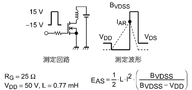
図 8.16 測定回路/測定波形
