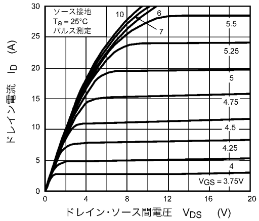
図 8.2 I_D - V_{DS}
