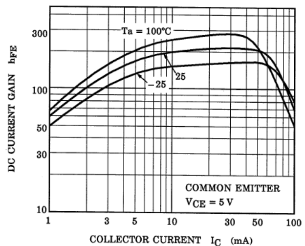
Fig. 10.18 RN1906FE h_{FE}-I_C
