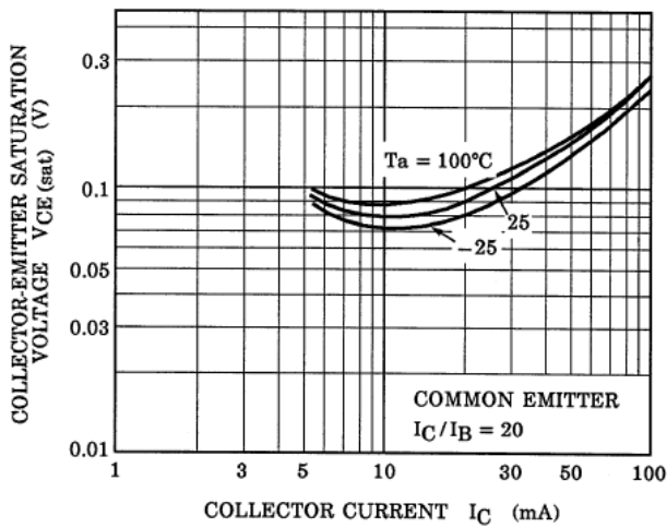
Fig. 10.19 RN1401 V_{CE(sat)}-I_C
