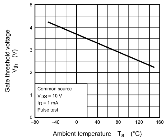
Fig. 8.10 V_{th} - T_a
