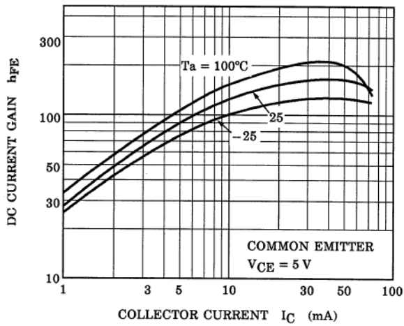
Fig. 10.15 RN1103 h_{FE}-I_C
