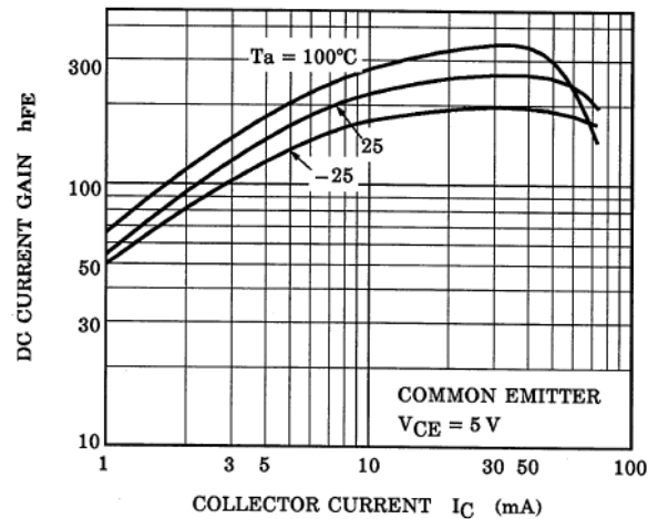
Fig. 10.16 RN1104 h_{FE}-I_C
