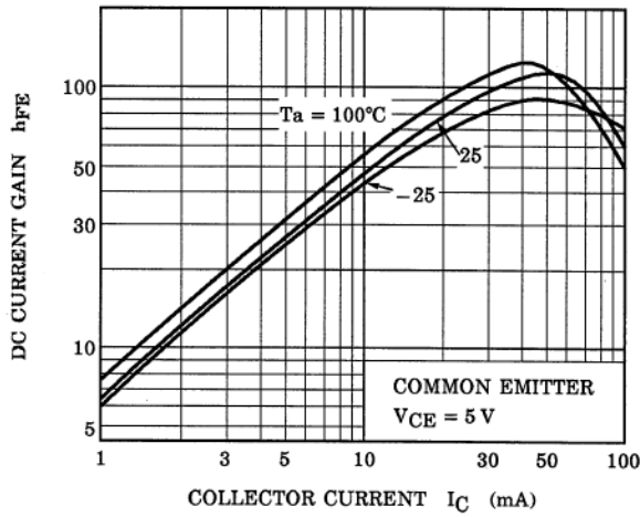
Fig. 10.13 RN1101 h_{FE}-I_C
