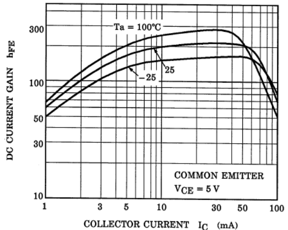
Fig. 10.18 RN1106 h_{FE}-I_C
