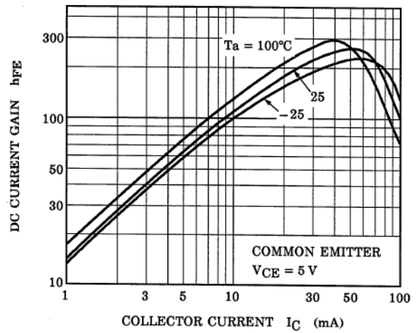
Fig. 10.14 RN1102 h_{FE}-I_C
