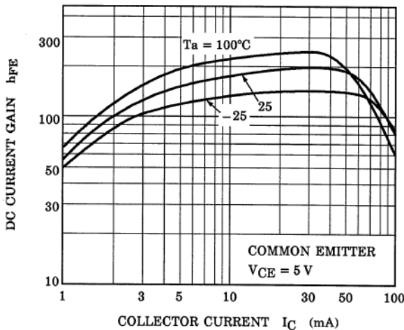
Fig. 10.17 RN1105 h_{FE}-I_C
