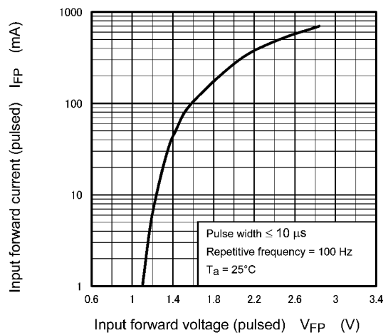
Fig. 11.6 I_{FP} - V_{FP}
