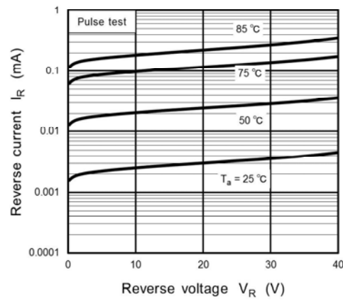
Fig. 9.2 I_R - V_R
