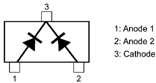
TBAT54C
