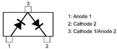
TBAT54S
