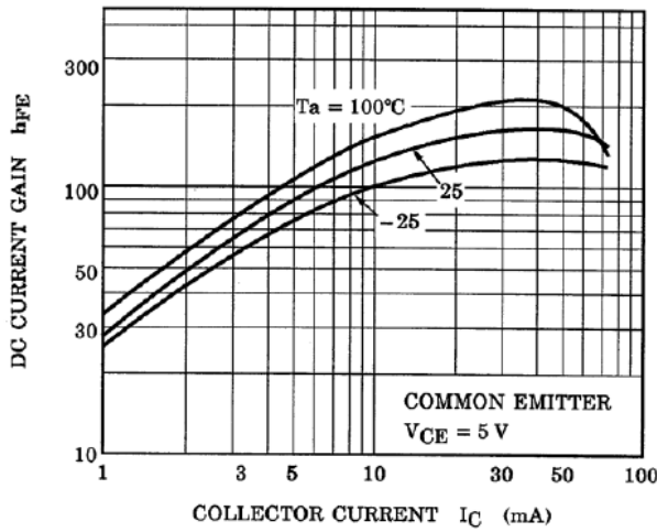
Fig. 10.15 RN1303 h_{FE}-I_C
