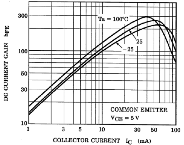
Fig. 10.14 RN1302 h_{FE}-I_C
