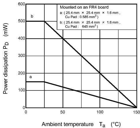
Fig. 7.11 P_D - T_a
