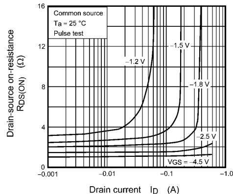
Fig. 7.6 R_{DS(ON)} - I_D
