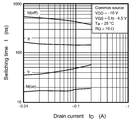
Fig. 7.10 t - I_D
