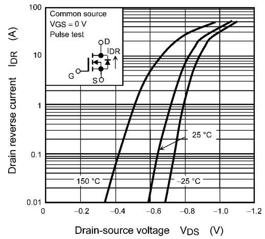
Fig. 8.8 I_{DR} - V_{DS}
