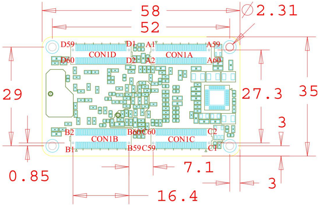
图 7 核心板机械尺寸图（顶层透视图）
