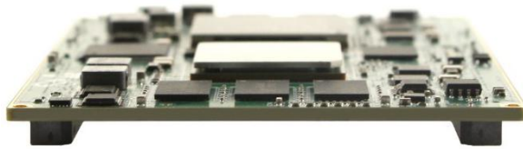
图 4 核心板侧视图
