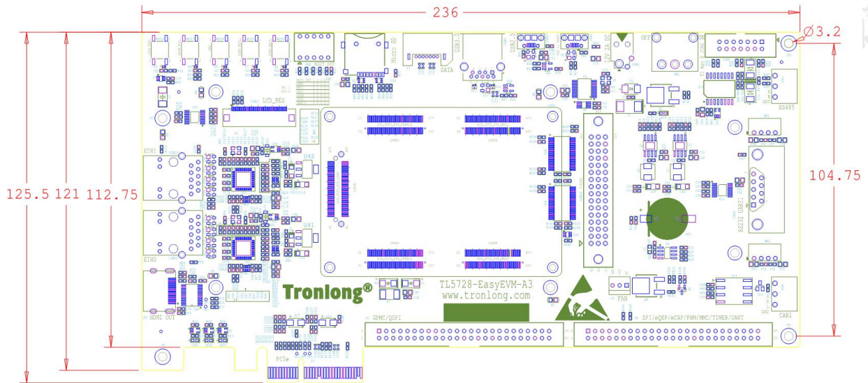
图 12 评估底板机械尺寸图
