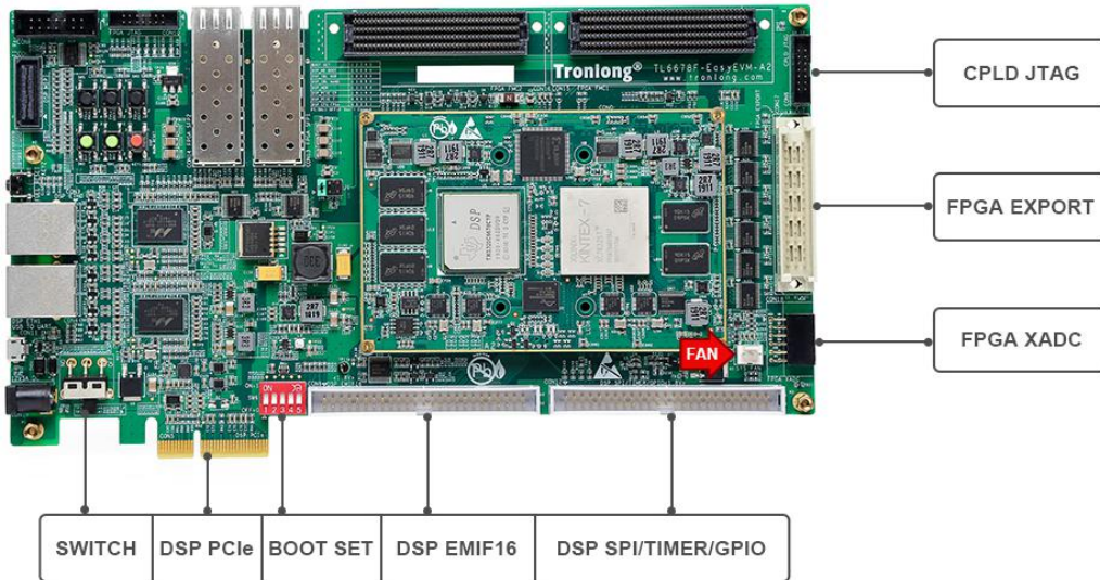
图 9 评估板硬件资源图解 2
