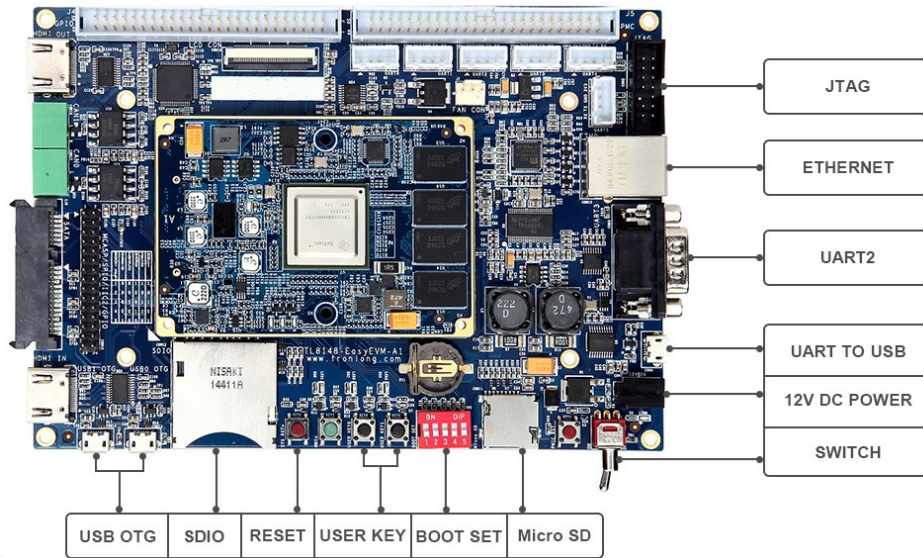
图 10 开发板硬件资源图解 2
