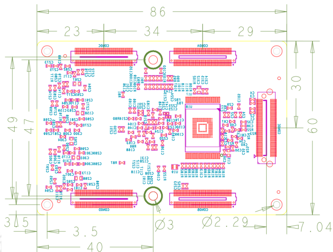
图 11 核心板机械尺寸图
