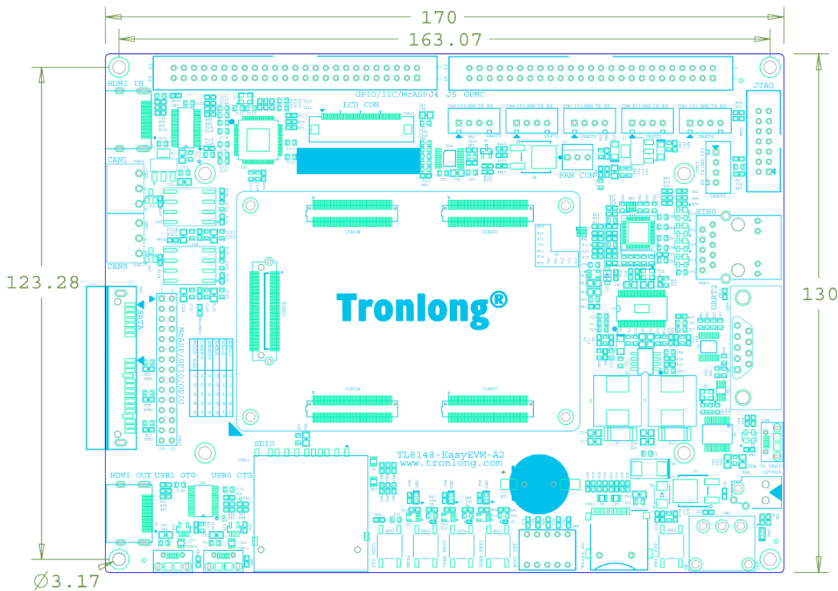
图 12 开发板机械尺寸图
