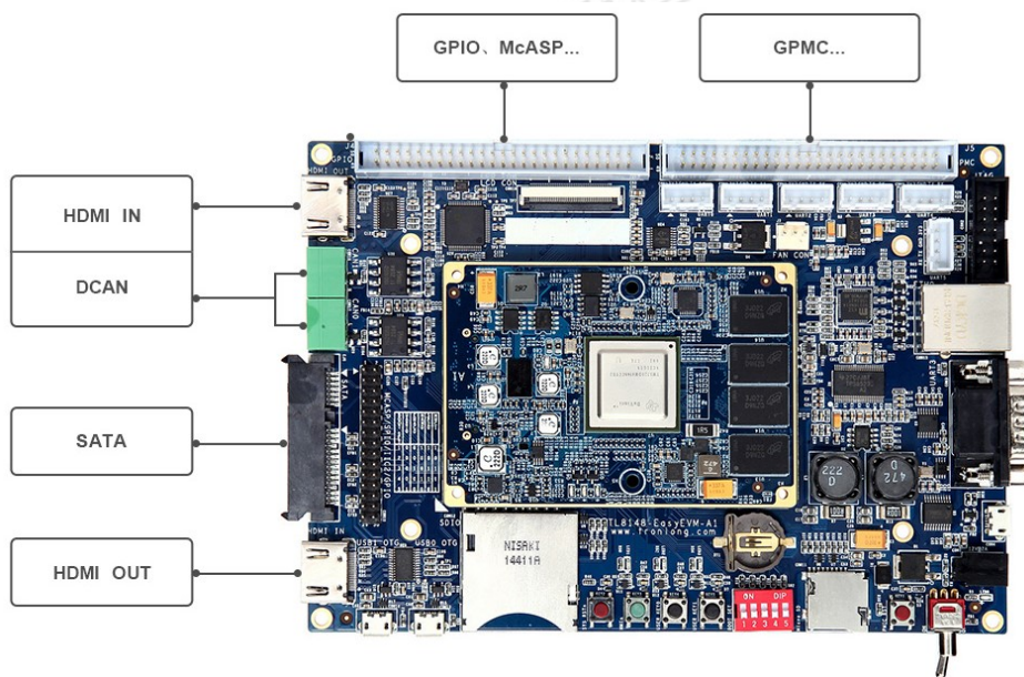
图 9 开发板硬件资源图解 1
