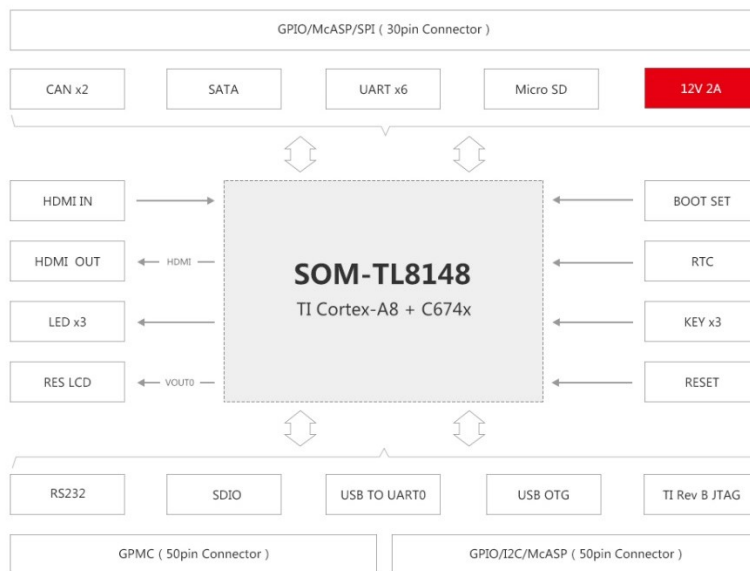
图 8 开发板硬件框图
