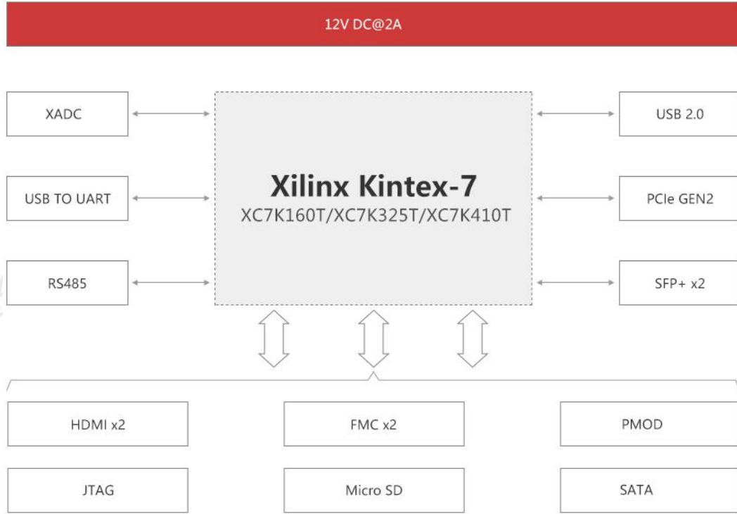
图 7 评估板硬件框图
