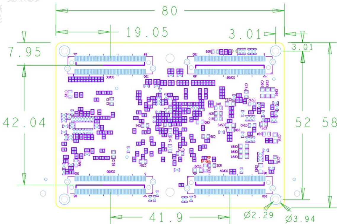
图 10 核心板机械尺寸图（顶层透视图）
