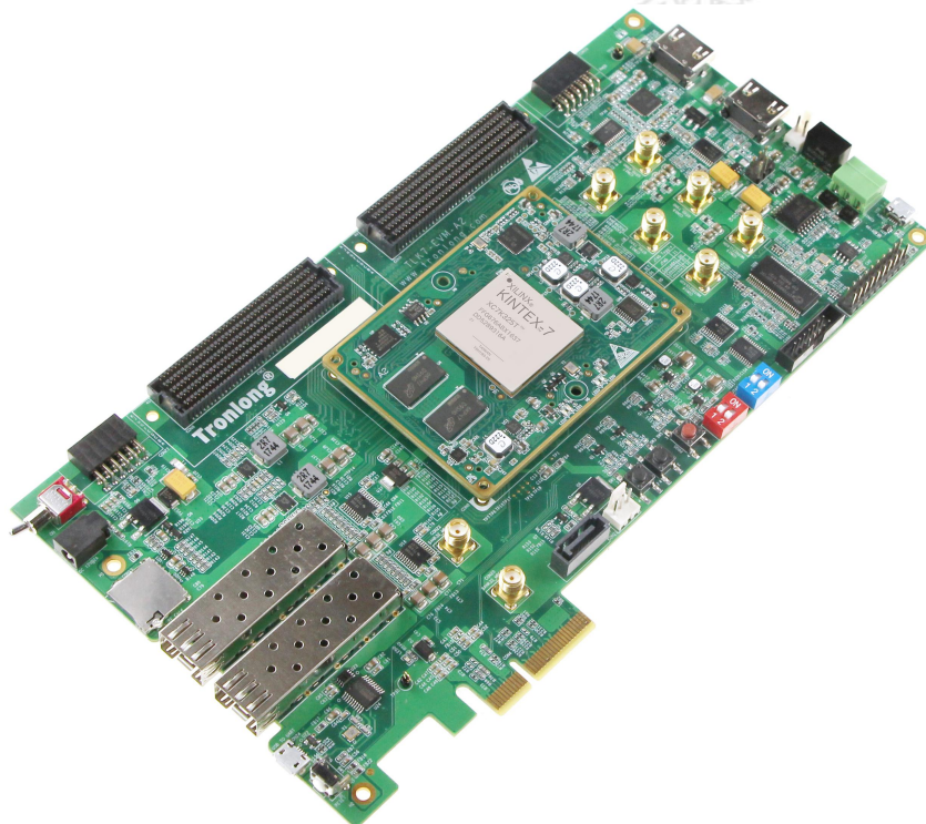
图 2 评估板斜视图
