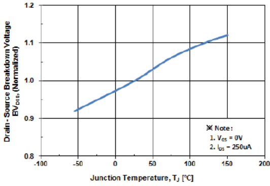
Fig. 7 BV_{DSS} - T_J
