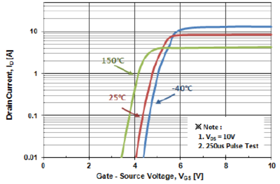
Fig. 2 I_D - V_{GS}
