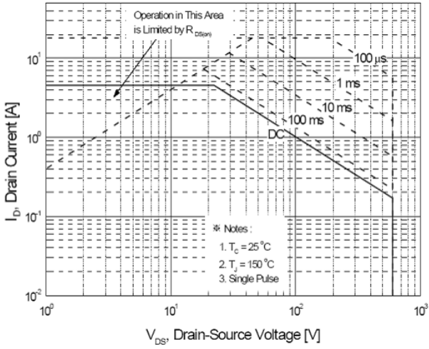
图 6-1 5N65(TO-220)
