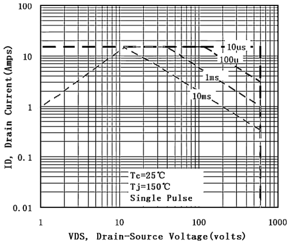
图 6-1 4N60 (TO-220)
