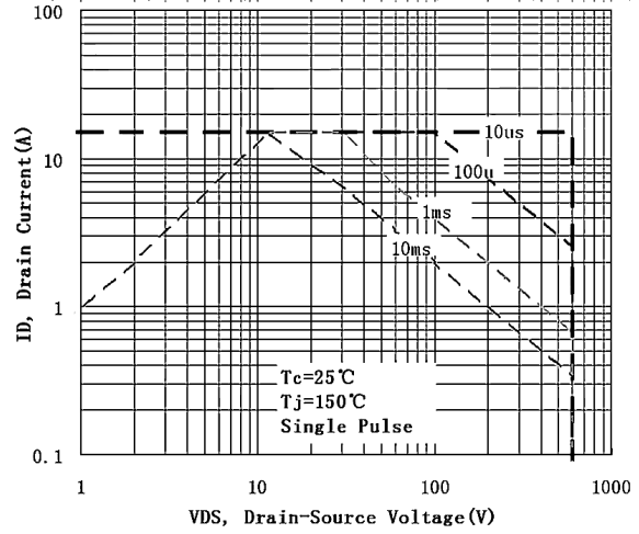
图 6-2 4N60(TO-220F)
