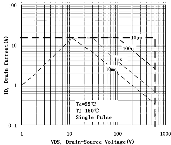
图 6-2 4N65(TO-220F)
