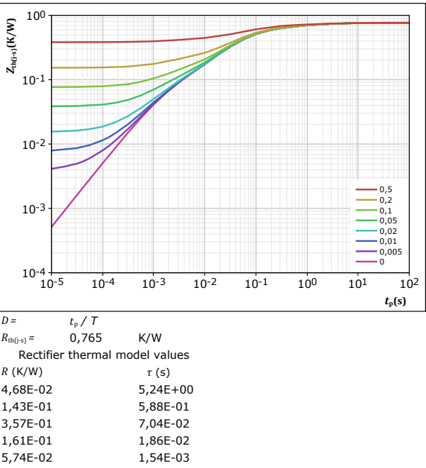
figure 20. Rectifier
