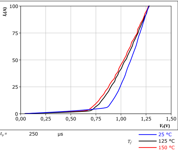
figure 19. Rectifier
