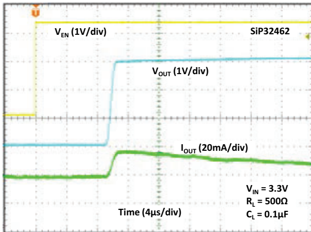
Fig. 32 - Turn-on Time
