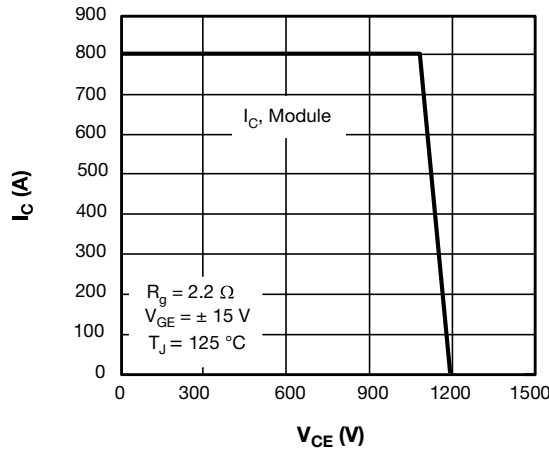
Fig. 5 - RBSOA
