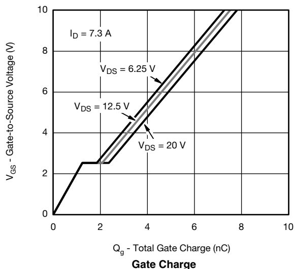
I_D = 7.3\text{ A} V_{DS} = 6.25\text{ V} V_{DS} = 12.5\text{ V} V_{DS} = 20\text{ V} Gate Charge
